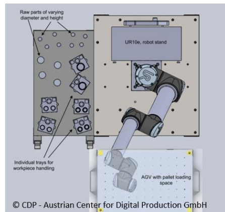
Abbildung 1: Beschreibung und Layout der Adaptive Loading Station
