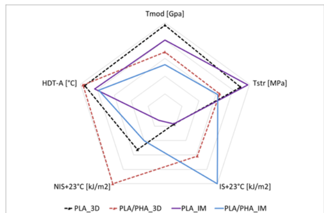
Für Experten: Eigenschaften von PLA und PLA/PHA; spritzgegossene (IM) und 3D-FLM gedruckte (3D) Teile.
