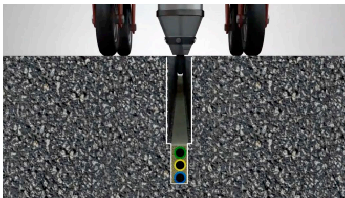
Abbildung 38: Aufbau Nano-Trench
