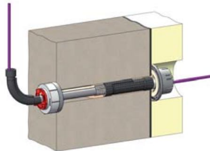
Abbildung 46: Mauerdurchführung
