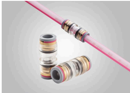
Abbildung 34: Steckmuffen
