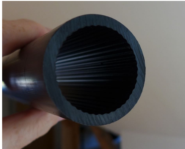
Abbildung 25: Kabelschutzrohr DA50 innen gerieft
