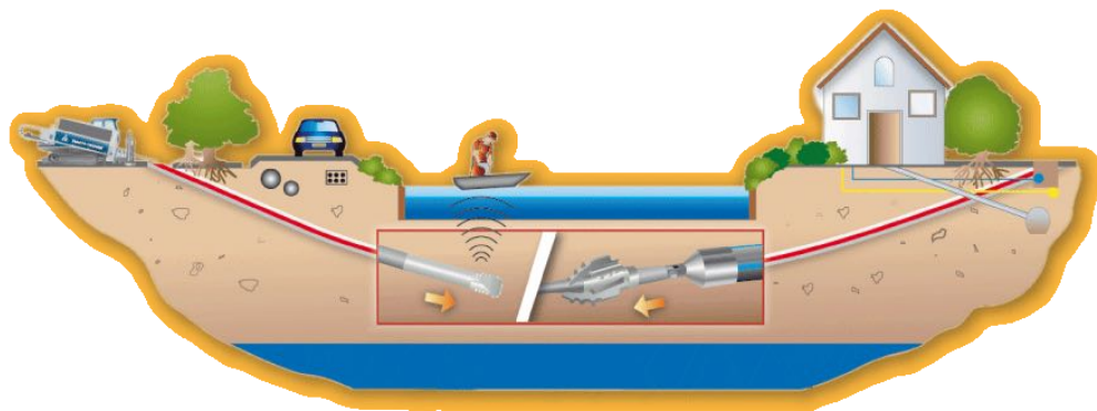
Abbildung 44: Horizontalspülbohrverfahren
