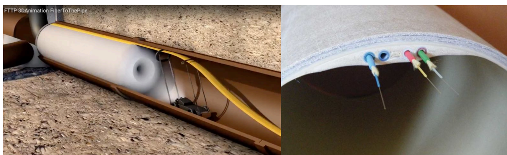
Abbildung 41: LWL-Verlegung durch Aufkleben eines Filzstreifens
