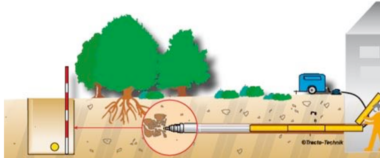
Abbildung 42: Prinzip Erdrakete
