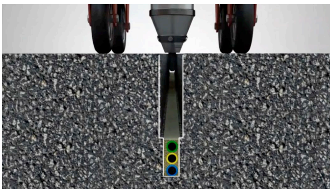
Abbildung 38: Aufbau Nano-Trench
