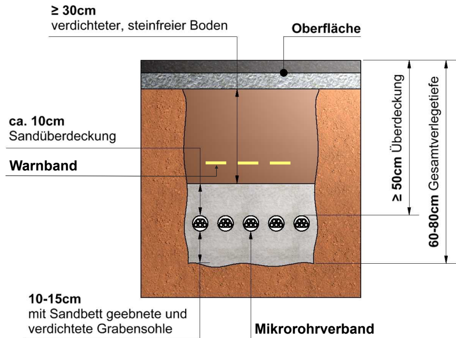
Abbildung 35: Typischer Einbau von Mikrorohrverbänden
