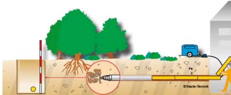
Abbildung 40: Prinzip Erdrakete
