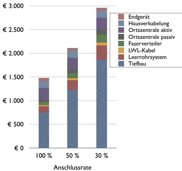
Abbildung 10: Investitionskosten nach Anschlussrate
